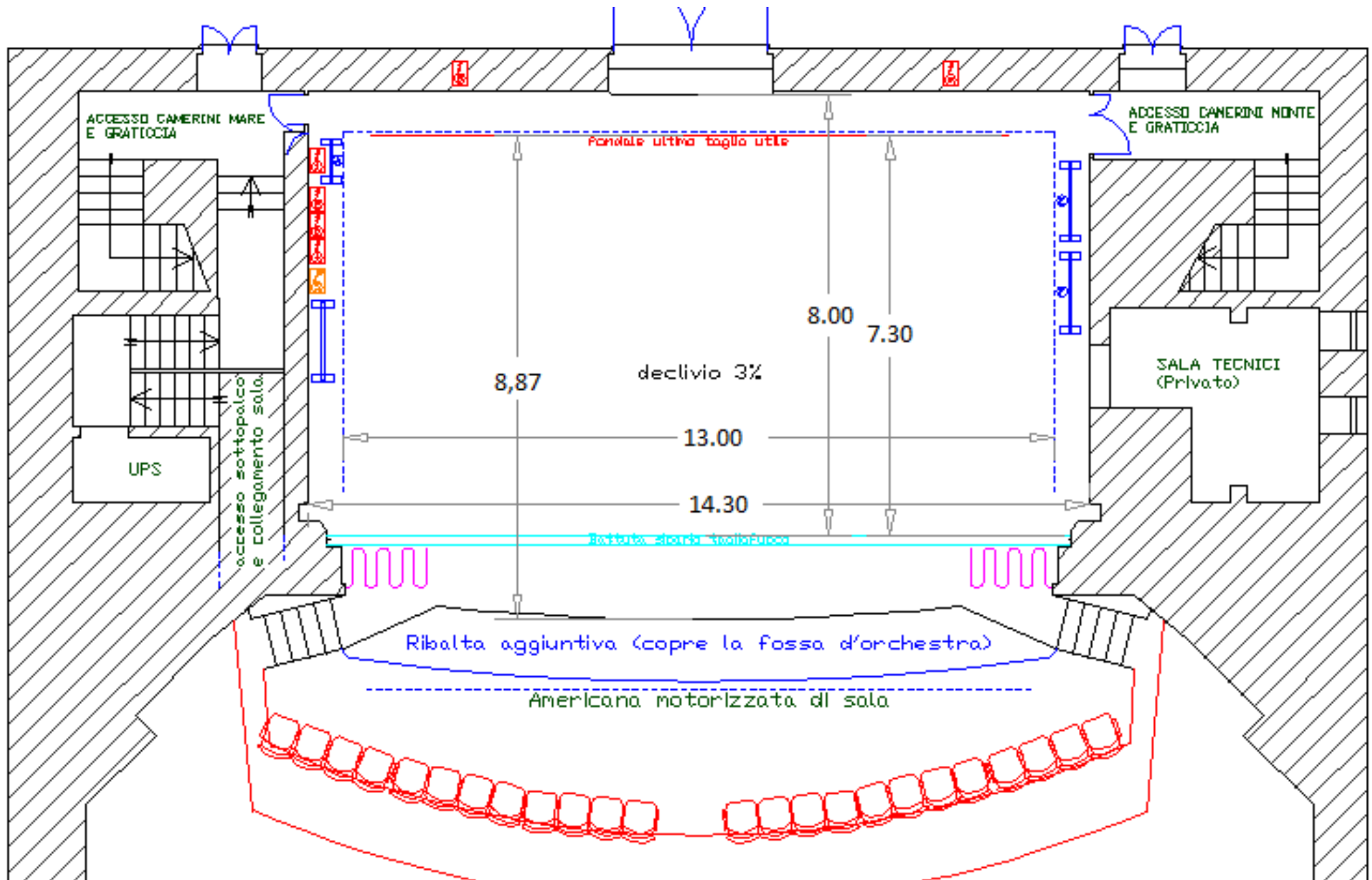
TEATRO COMUNALE TRAIANO - CIVITAVECCHIA – PIANTA PALCOSCENICO
